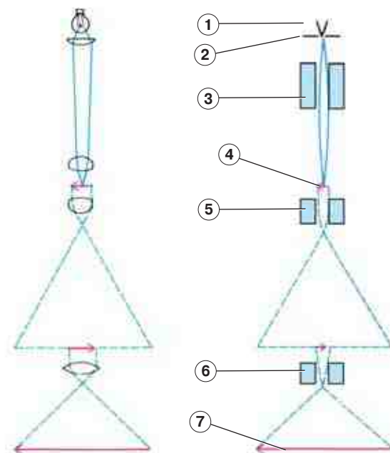
Рис. 1.20. Ход лучей в световом (слева) и электронном (справа) микроскопах [по М. Росс и Е. Рейтх]
