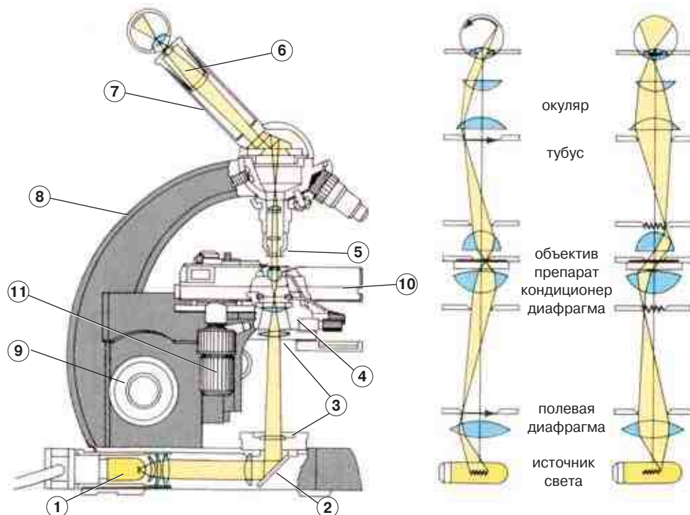
Рис. 1.1. Световой микроскоп и ход в нем лучей света [по М. Росс и Е. Рейтх]
